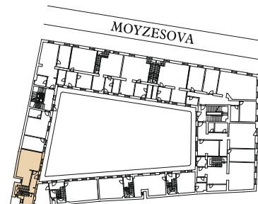
PÓDORYS 1. POSCHODIA
