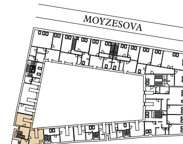
PÓDORYS PODKROVIA
